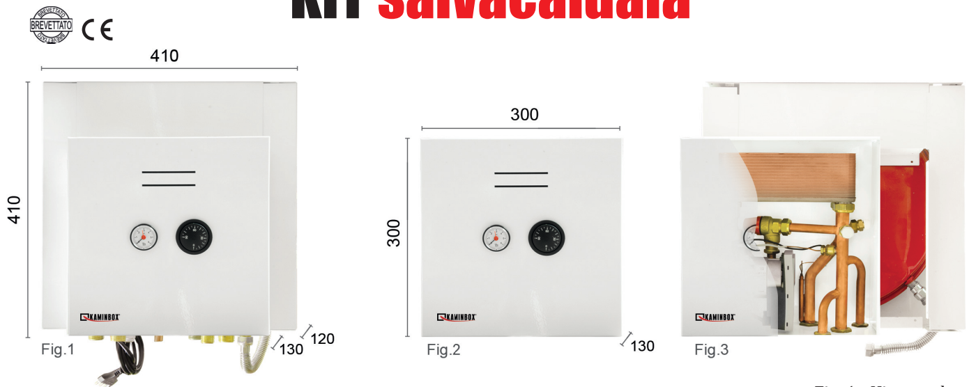
Fig. 1 - Kit completo Fig.2 - Kit escluso di vaso d'espansione Fig. 3 - Spaccato del kit completo
